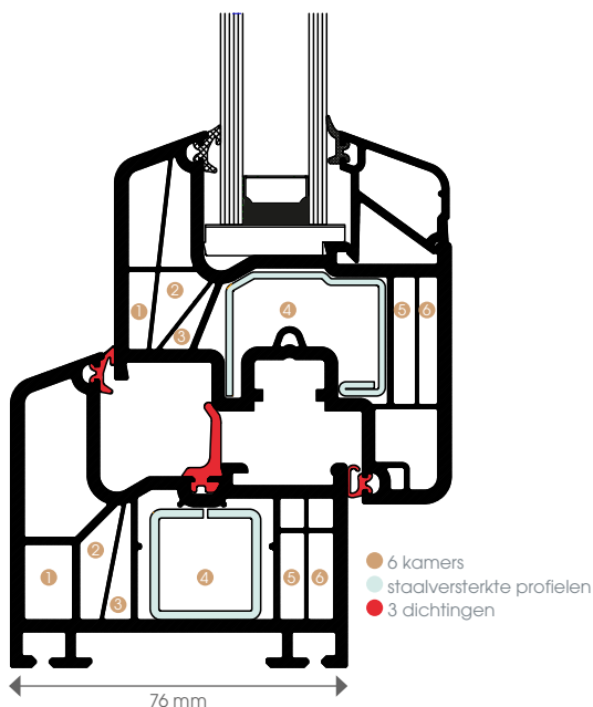
Fig. 1: staalverstevigingen, 3 dichtingen en 6 kamers
